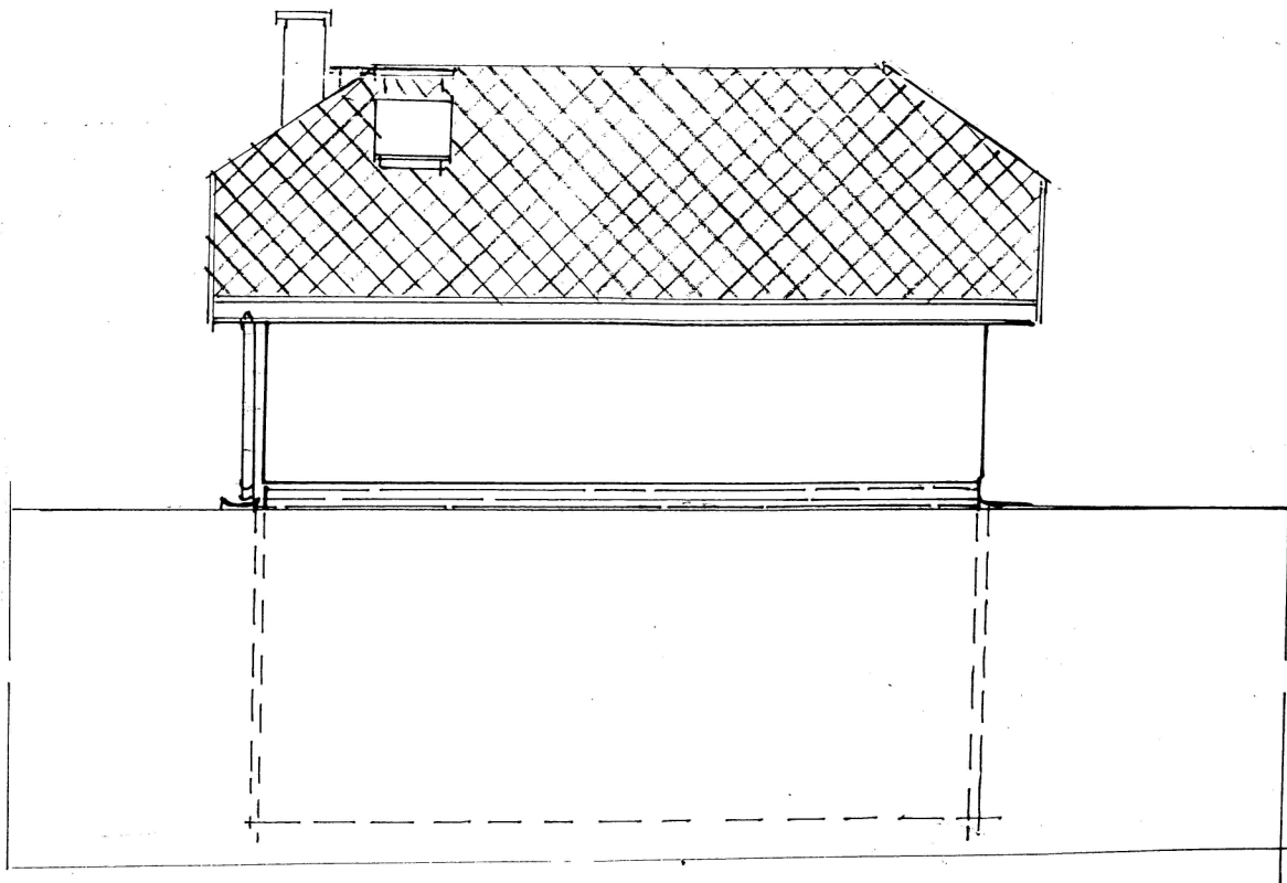
Elewacja południowa 1:100
