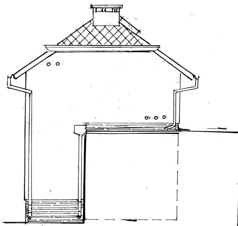
Elewacja zachodnia 1:100
